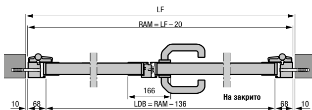
Странична врата с 2 крила и алуминиева блок-каса, профил тип 2 Монтаж в отвора
