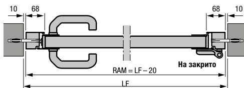
Странична врата с алуминиева блок-каса, профил тип 2 Монтаж в отвора
